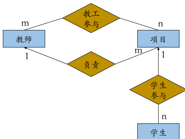
图 2.12: 基于业务描述的 ER 设计实例
