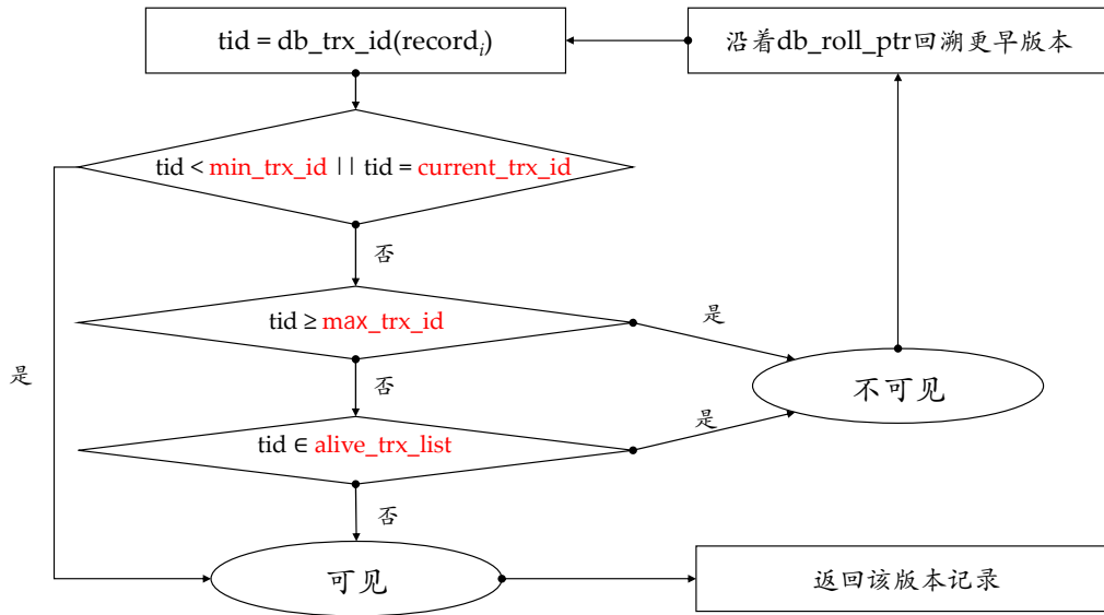
图 9.15: 可见性算法规则流程图
