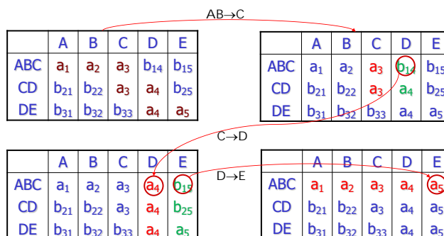
图 7.6: 无损连接分解判别算法示例
