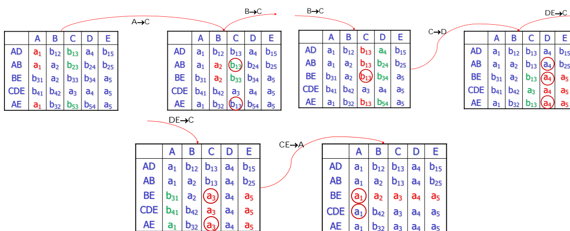
图 7.7: 无损连接分解判别算法示例
