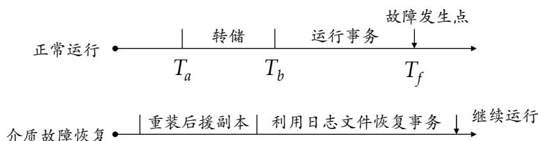
图 10.5: 介质故障恢复过程
