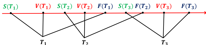
图 9.11: 有效性检查协议的例子
