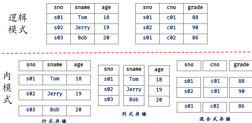
图 1.4: 数据库内模式的例子
