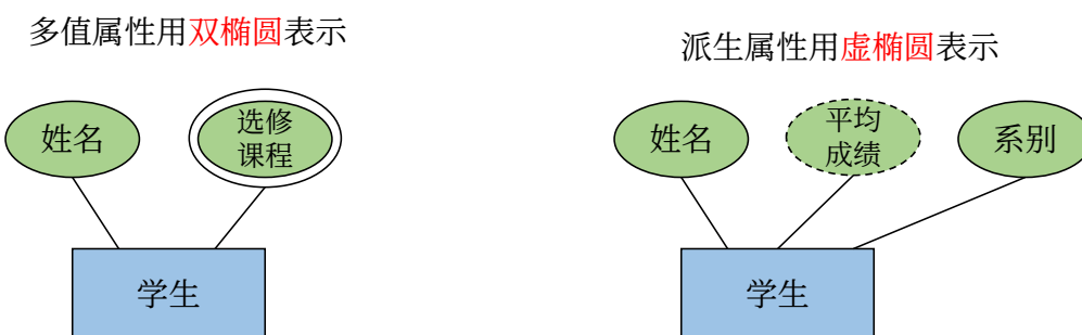
图 2.4: 多值属性和派生属性的表示
