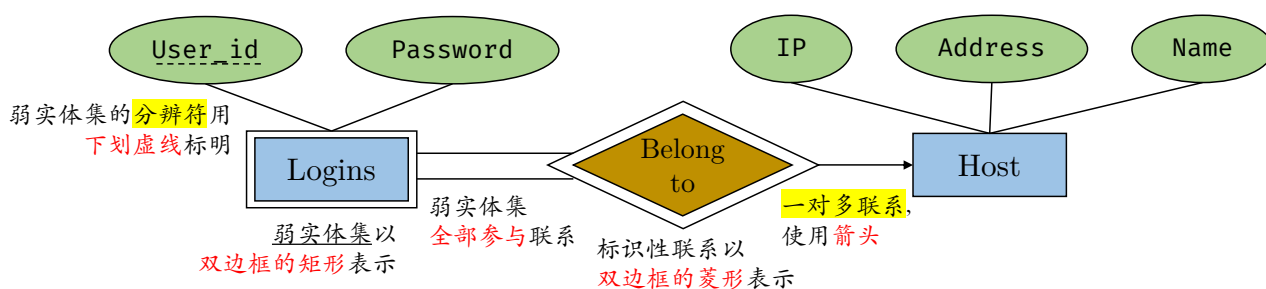
图 2.17: 弱实体集的 ER 表示
