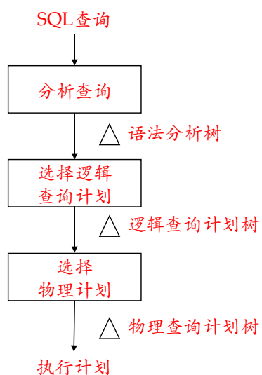
图 12.1: 查询处理步骤
