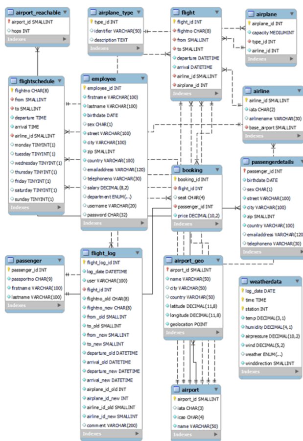
图 2.23: airportdb 的表结构
