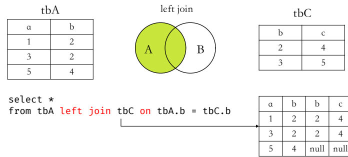
图 4.9: left join 示例
