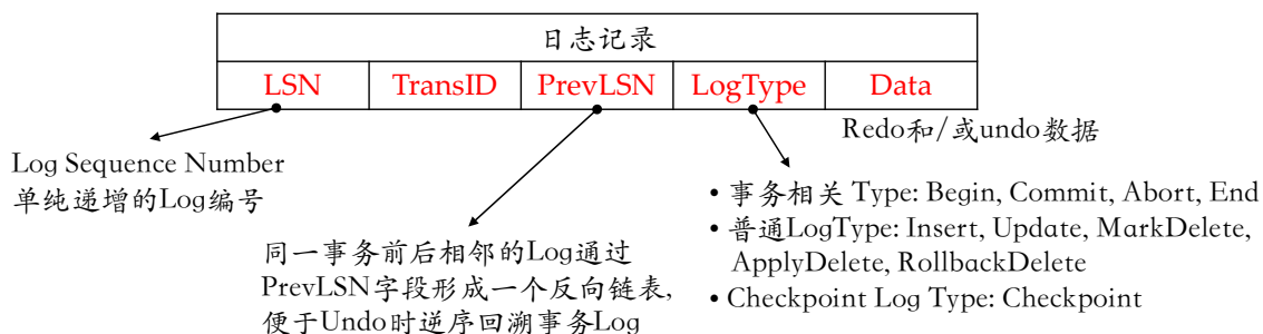
图 10.11: 日志记录结构
