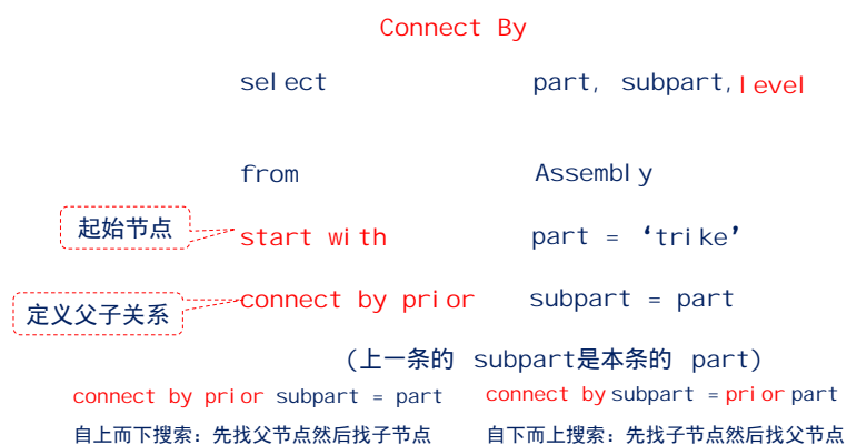
图 6.2: Oracle 中的递归查询
