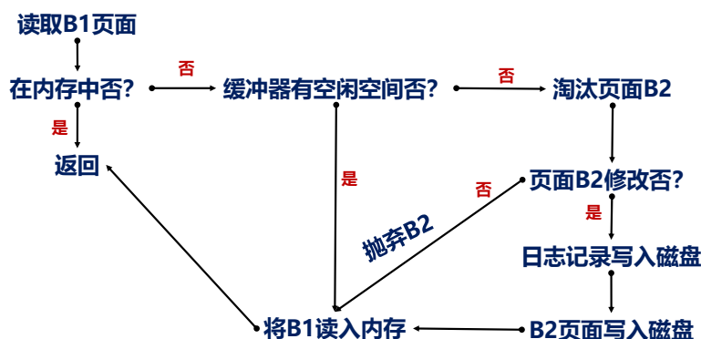
图 10.4: 读取一个页面的过程 (actually from 操作系统)
