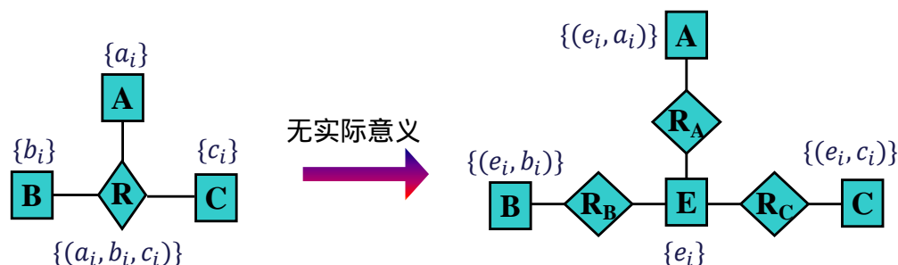
图 2.21: 无意义的转换
