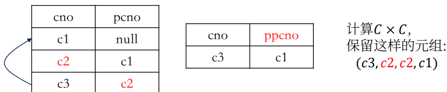
图 3.10: 先修课的先修课
