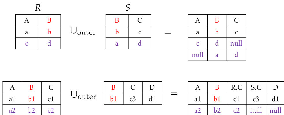
图 3.8: 外部并示意图
