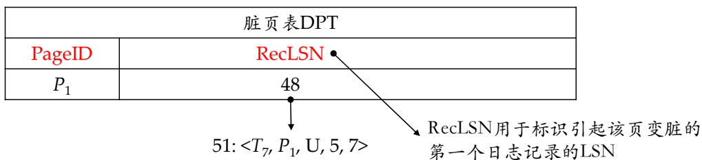
图 10.13: 脏页表结构
