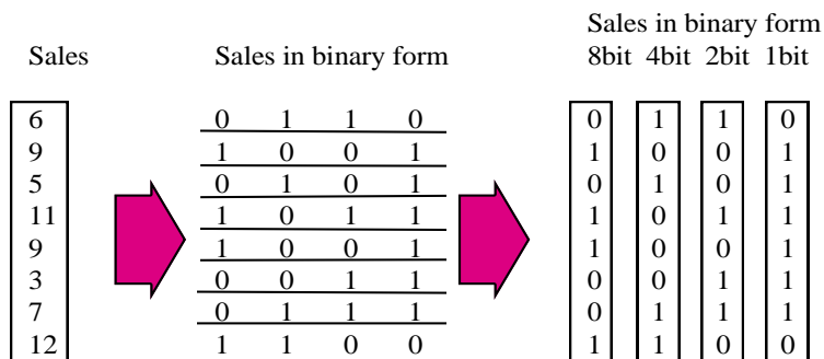
图 11.14: 位片索引
