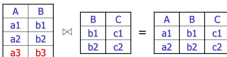
图 7.10: 悬挂元组
