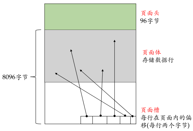
图 11.7: 基本页结构
