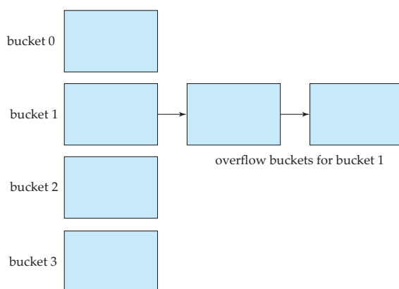
图 11.11: 溢出链
