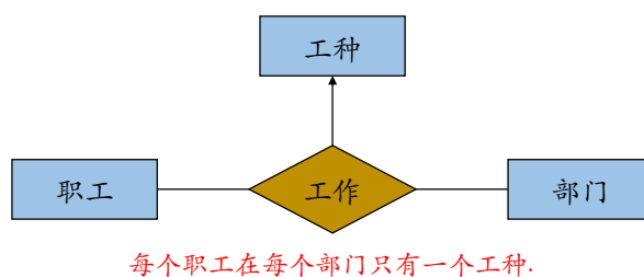
图 2.10: 多元联系
