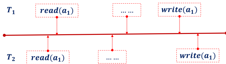
图 9.2: 转换死锁
