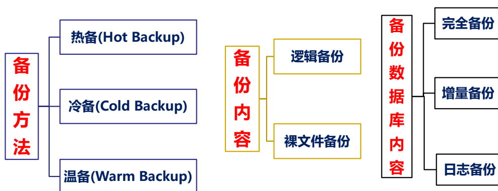
图 10.1: MySQL 备份
