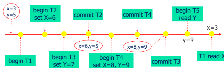
图 8.2: 快照隔离
