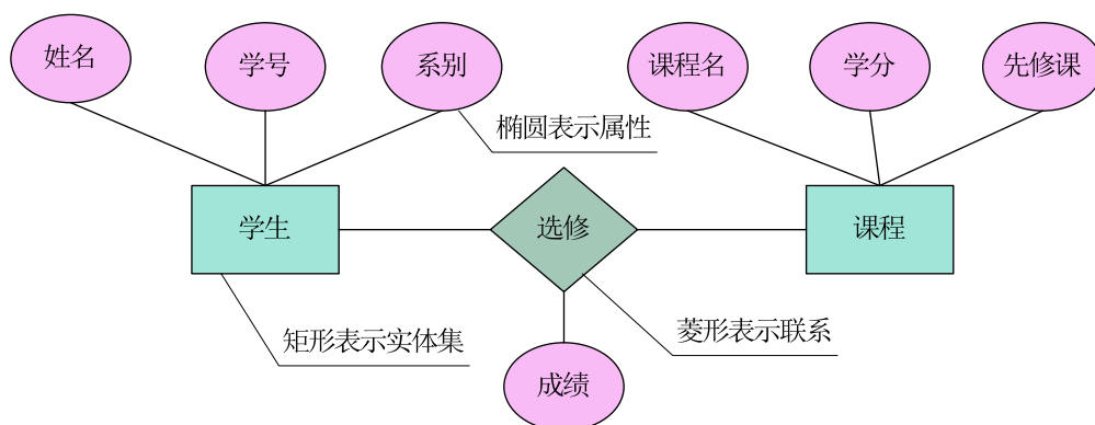
图 2.1: E-R 图
