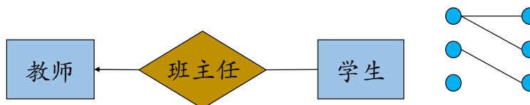
图 2.7: 一对多联系
