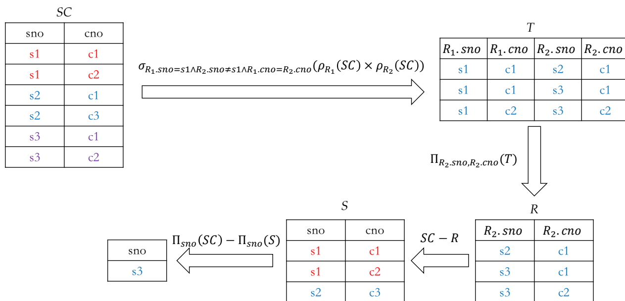
图 3.11: 问题解答
