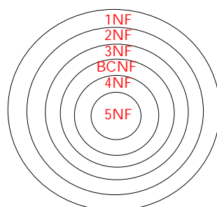
图 7.1: 范式
