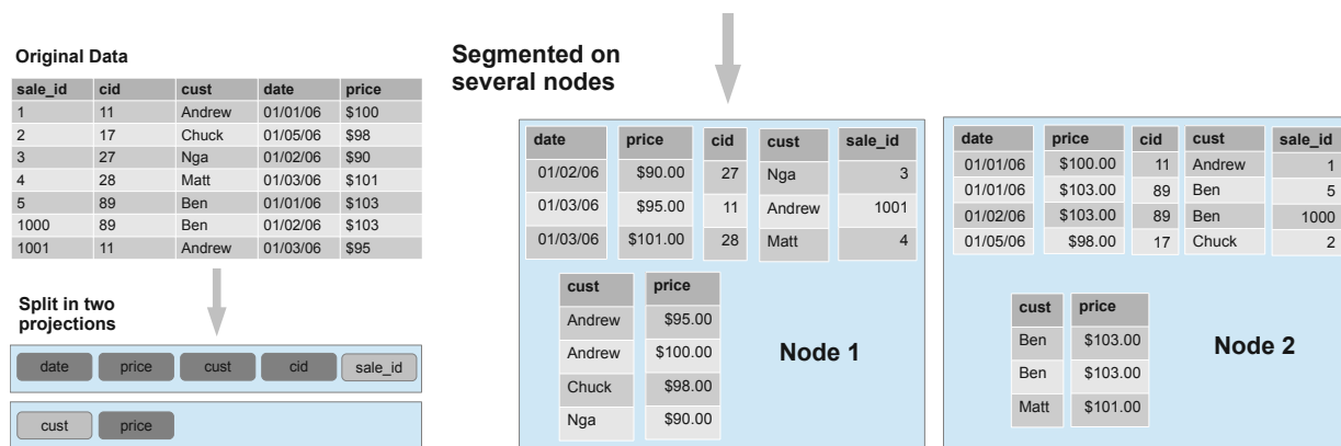
图 11.15: Vertica 的实现
