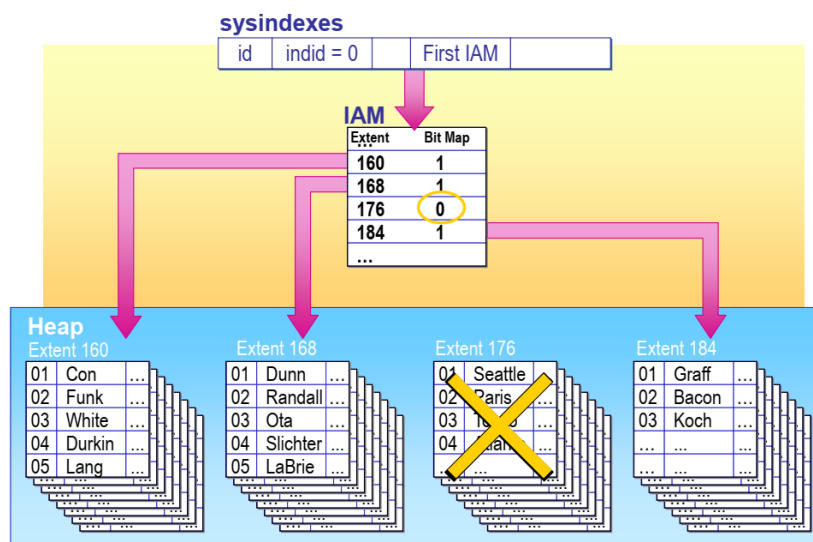
图 12.2: 堆上的表
