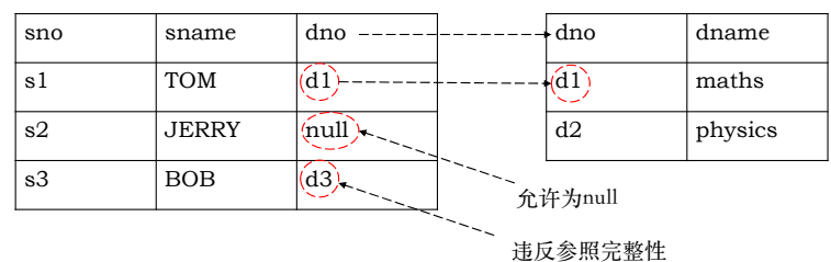
图 3.1: 参照完整性
