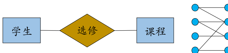
图 2.8: 多对多联系
