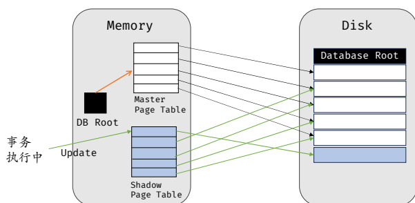
图 10.2: Shadow Paging: 正在修改的事务
