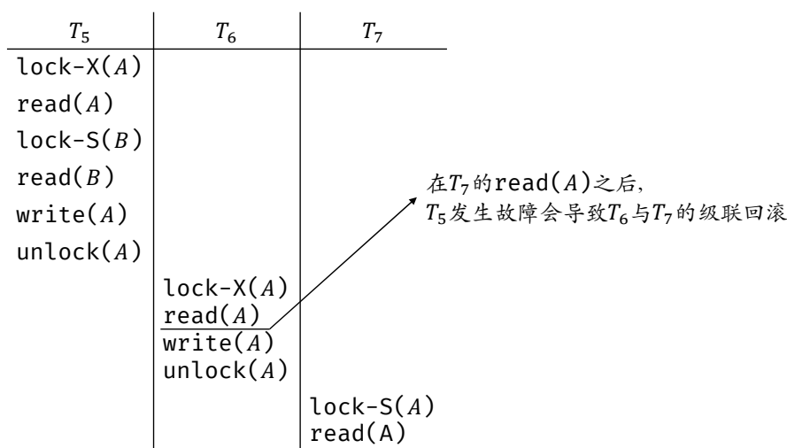
图 9.1: 2PL 的级联回滚
