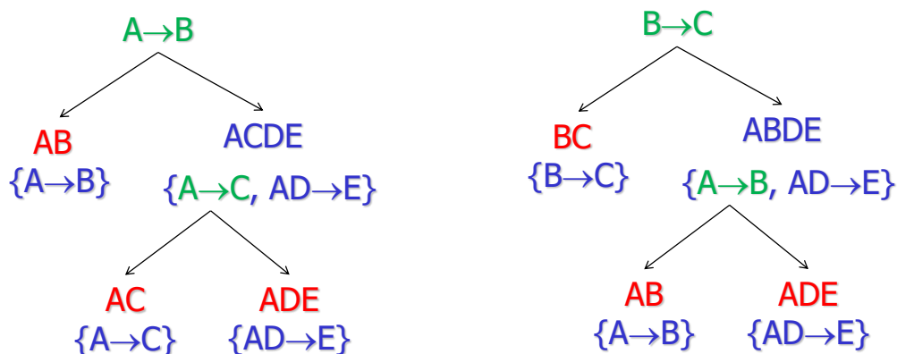
图 7.8: 达到 BCNF 无损连接分解算法
