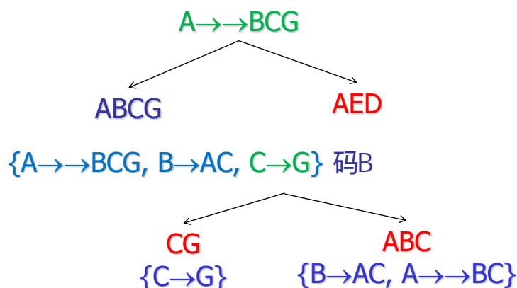
图 7.9: 达到 4NF 无损连接分解算法
