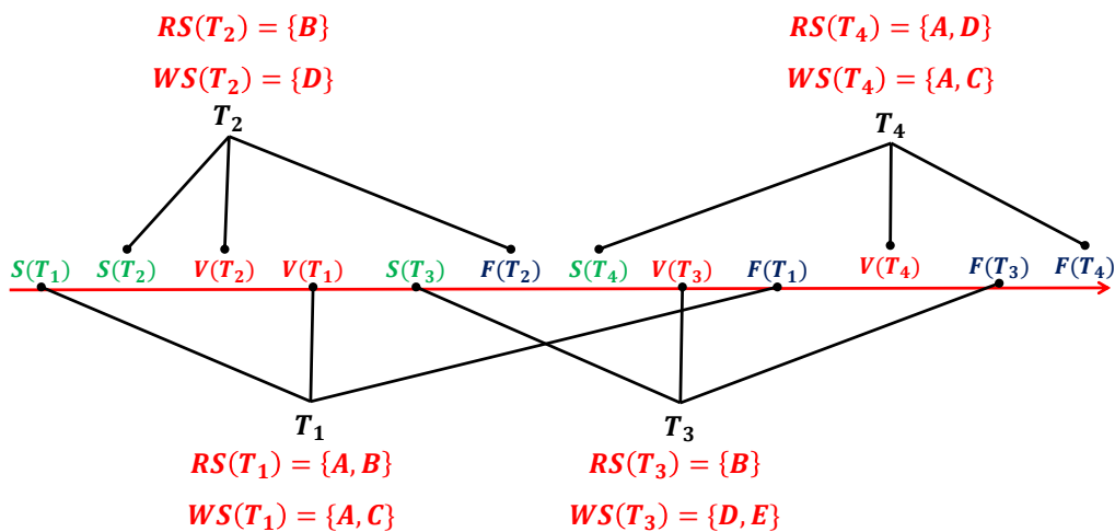
图 9.12: 有效性检查协议的另一个例子
