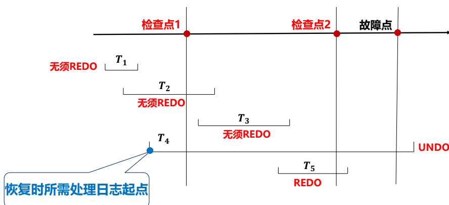
图 10.6: 检查点在系统故障恢复中的作用
