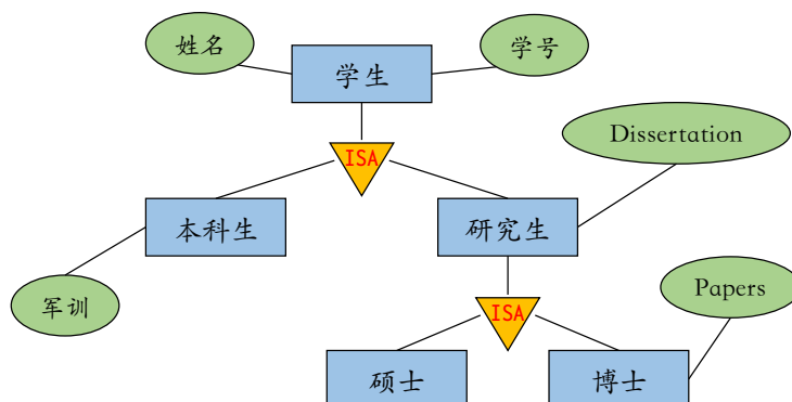
图 2.18: 特化的 ER 表示
