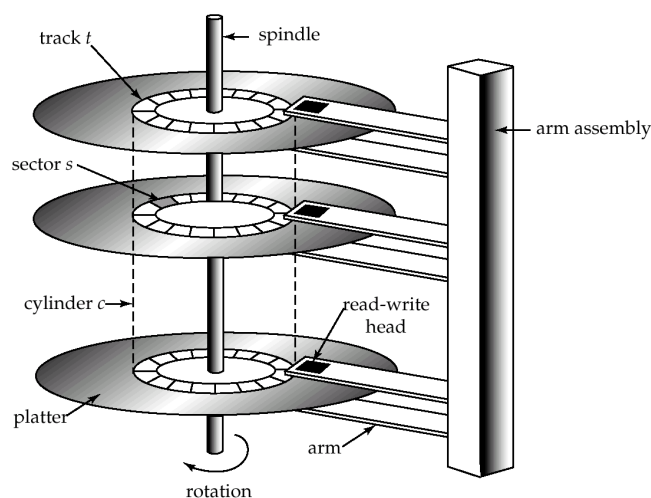
图 11.2: 磁盘的物理结构
