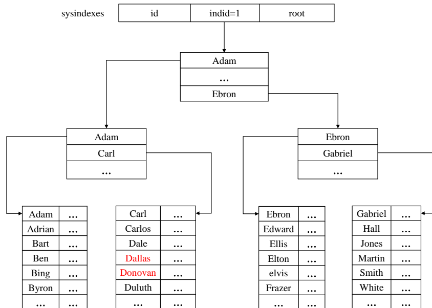
图 9.5: 码范围锁示例
