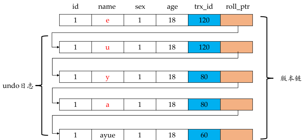
图 9.13: MySQL MVCC 实现: 数据行
