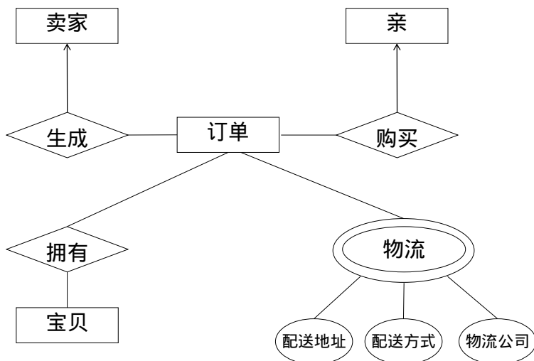
图 2.14: 由业务单据生成 ER 模型
