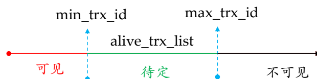
图 9.14: 可见性算法规则
