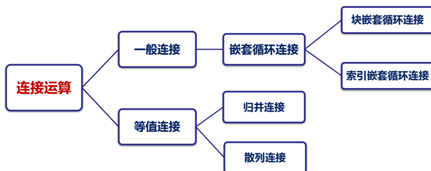
图 12.4: 实现各种逻辑运算的物理算子概览
