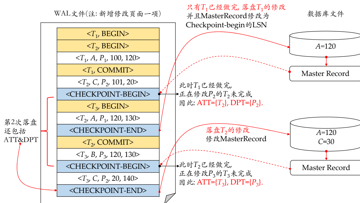
图 10.7: 模糊检查点的一个例子
