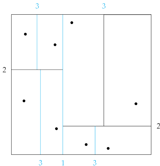
图 11.16: k-d 树的例子
