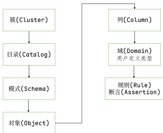
图 4.1: 标准 SQL 中的数据定义对象
