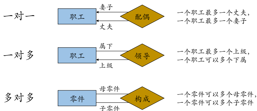
图 2.9: 一个实体集内的递归联系
