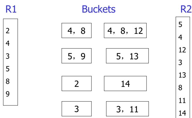
图 12.5: 散列连接示例
