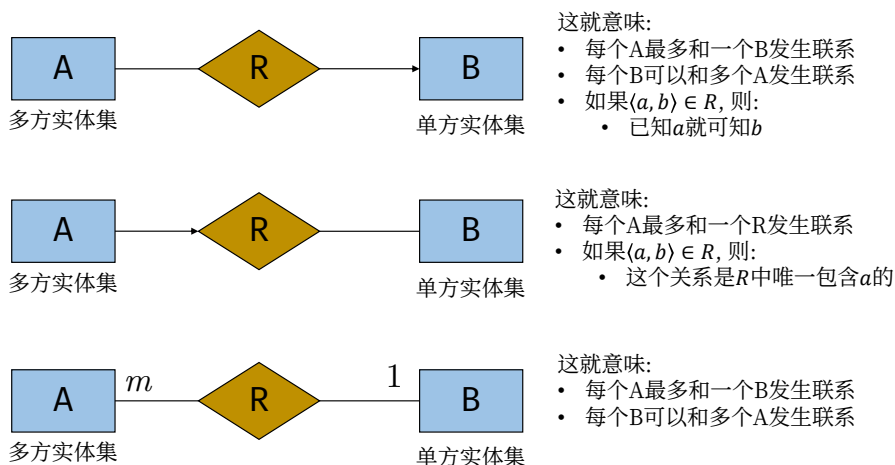
图 2.5: 联系种类在 E-R 图中的表示
