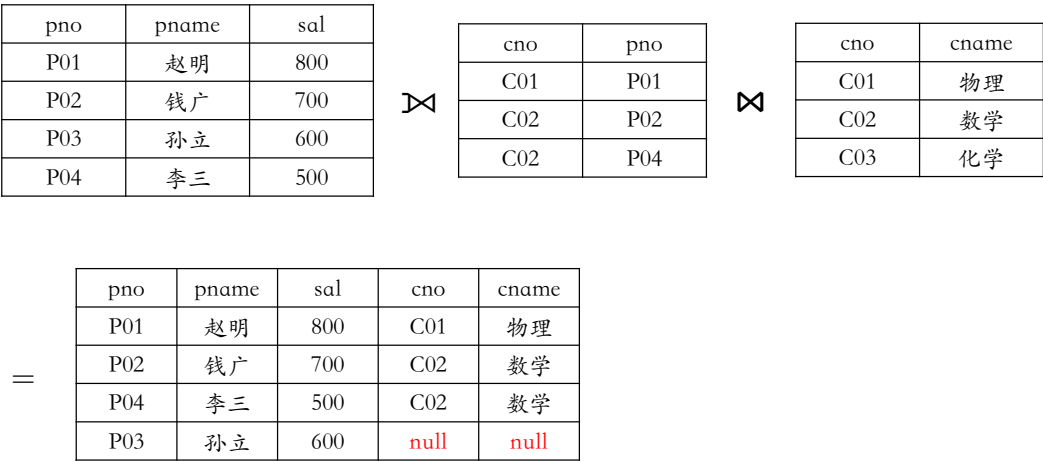
图 3.5: 左外连接示意图
