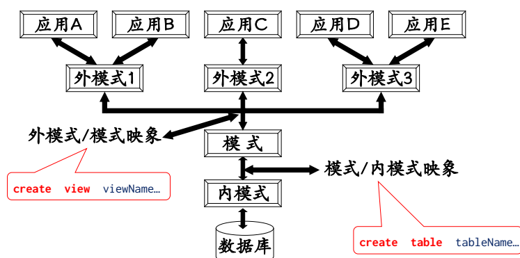
图 1.3: 数据库的三种模式
