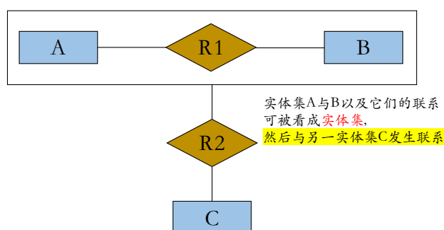
图 2.20: 聚集的 ER 表示
