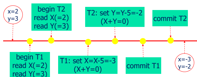
图 8.3: 快照隔离中的不一致现象
