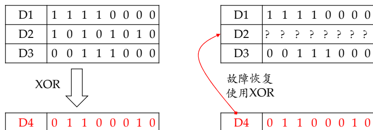
图 11.4: RAID 3: 位交叉奇偶校验
