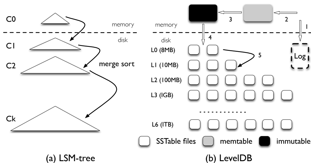
图 11.19: LSM 树的结构
