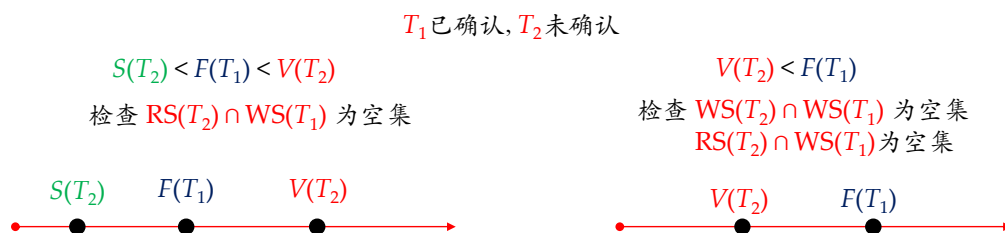
图 9.10: 有效性协议的检查条件
