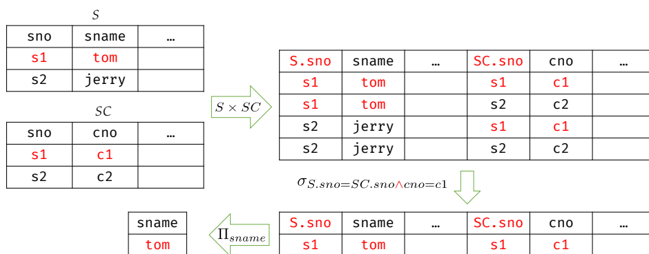
图 3.3: 笛卡尔积的使用
