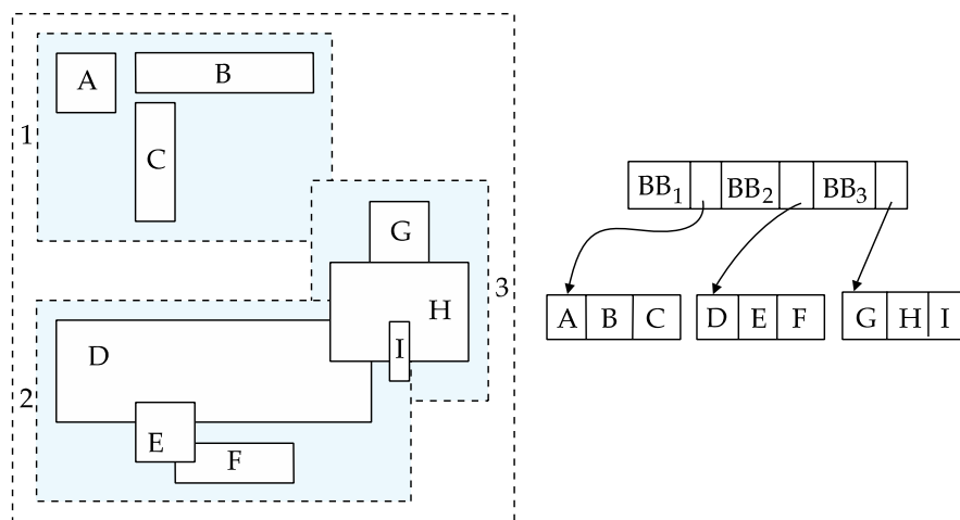
图 11.18: R 树的例子
