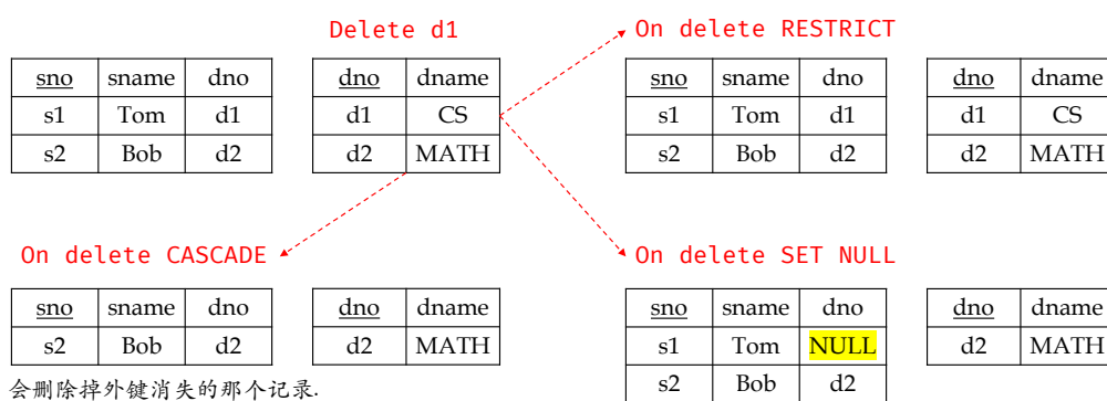
图 5.2: 外键的三种定义
