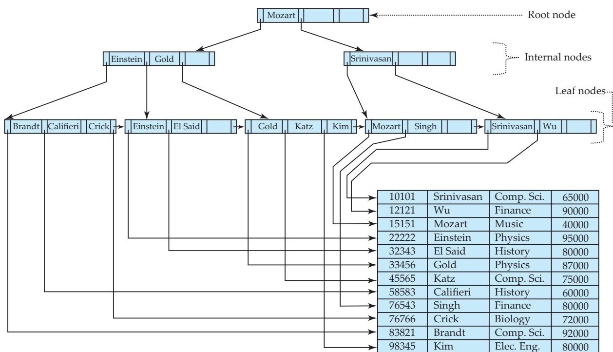
图 11.10: n = 4 的时候的 B+ 树
