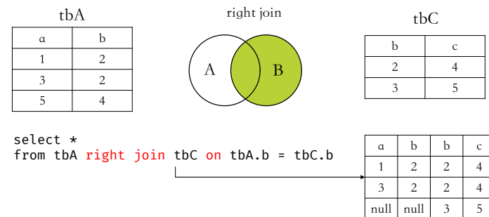
图 4.10: right join 示例
