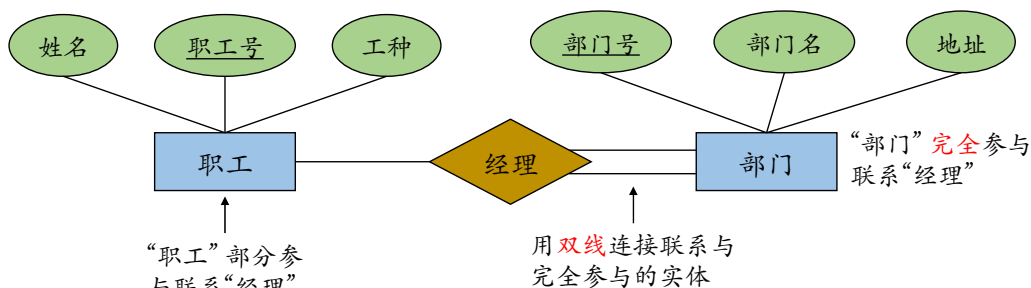
图 2.15: 参与的 ER 图表示
