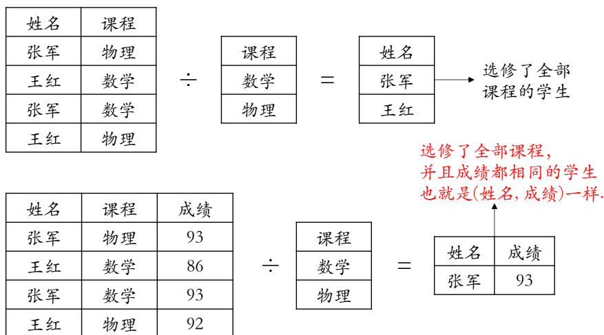
图 3.9: 对于除运算中的被除关系要正确投影
