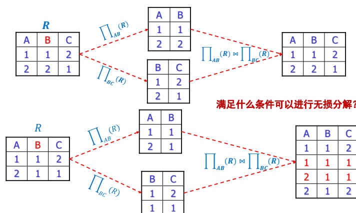
图 7.5: 无损分解的例子
