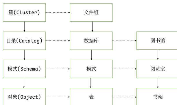
图 4.2: 实际数据库 (SQL Server) 中的定义对象
