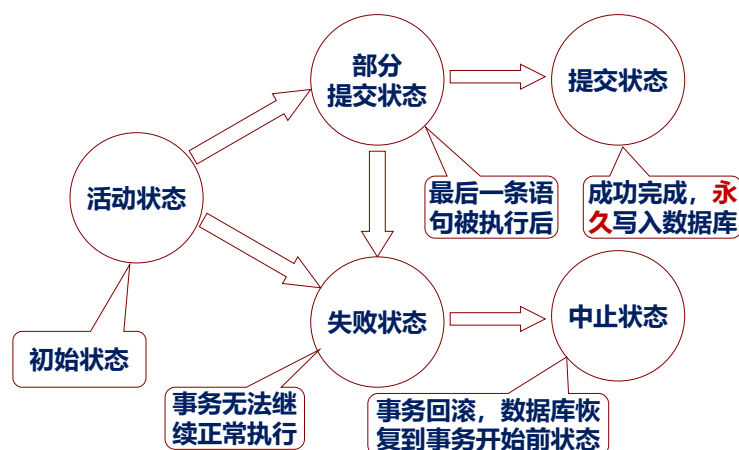
图 8.1: 事务生命周期图
