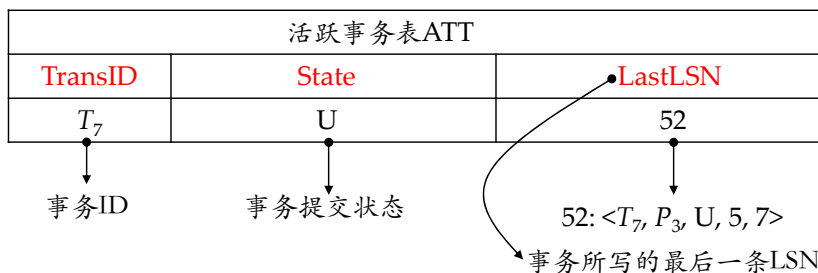
图 10.14: 活跃事务列表 (ATT) 结构
