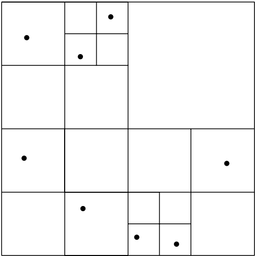
图 11.17: 四叉树的例子
