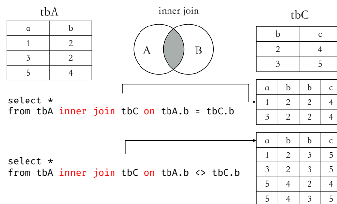
图 4.8: inner join 示例
