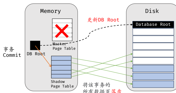
图 10.3: Shadow Paging: 事务 Commit
