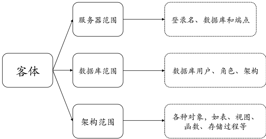
图 5.3: 客体分类
