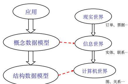
图 1.1: 数据模型
