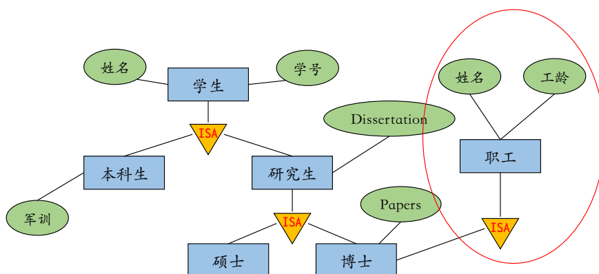
图 2.19: 格结构
