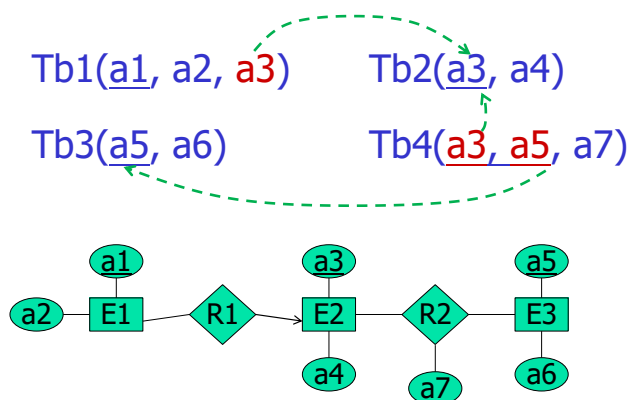
图 2.22: 逆向转换
