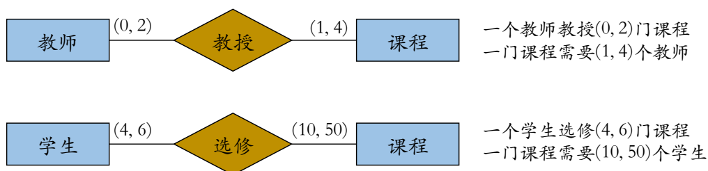
图 2.11: 联系的势
