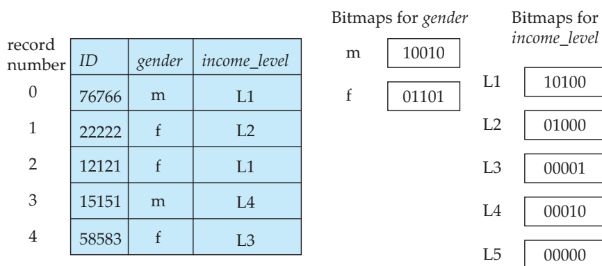
图 11.13: 位图索引
