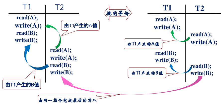
图 8.4: 视图等价
