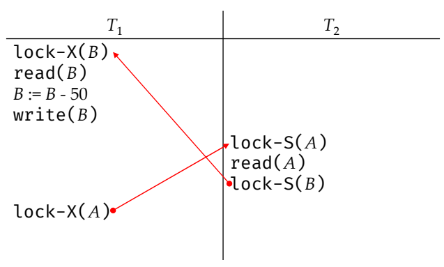
图 9.7: 死锁
