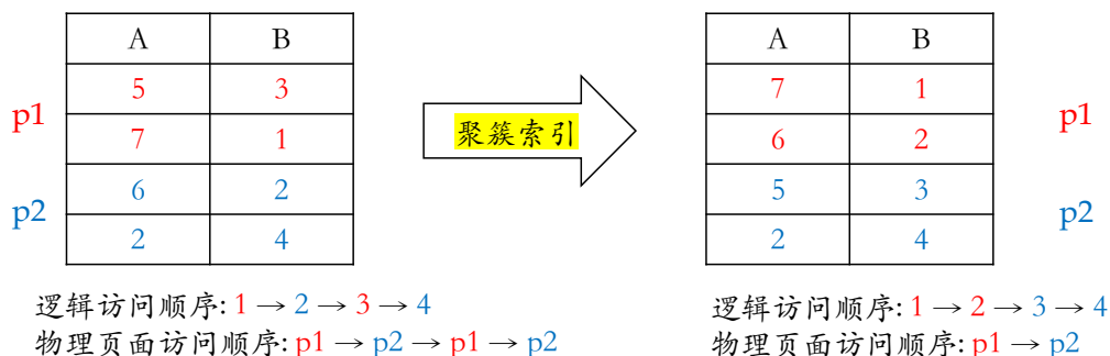
图 4.4: 聚簇索引
