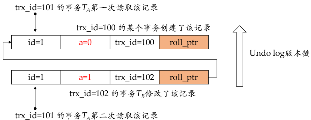
图 9.17: MVCC 读取
