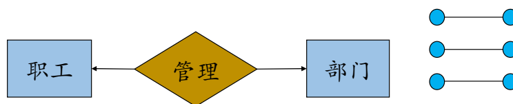
图 2.6: 一对一联系
