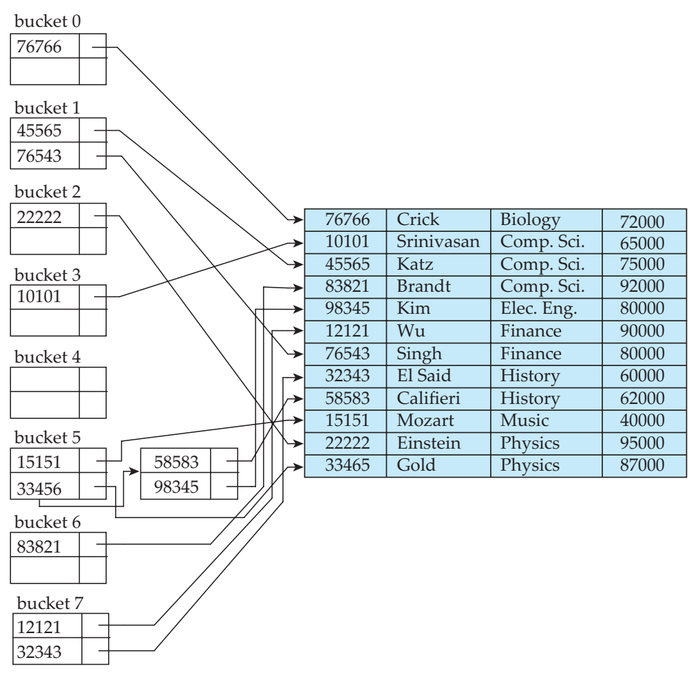
图 11.12: 散列索引
