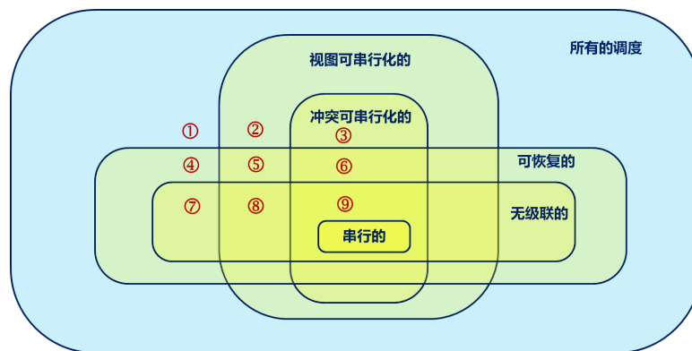
图 8.6: 调度类型
