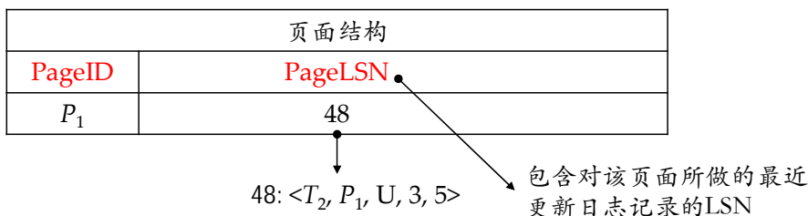
图 10.12: 页面结构
