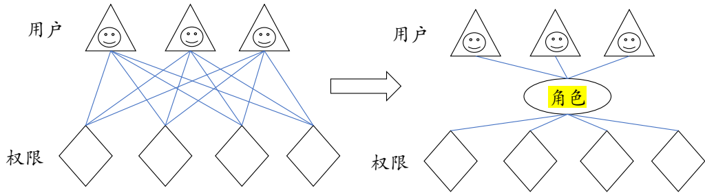
图 5.4: 数据库角色
