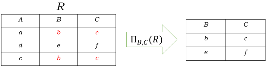
图 3.2: 投影运算要去掉相同的行
