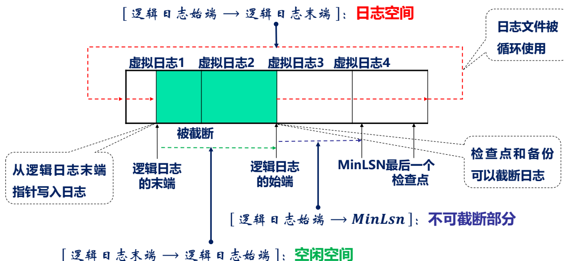
图 10.8: MinLSN 计算示例
