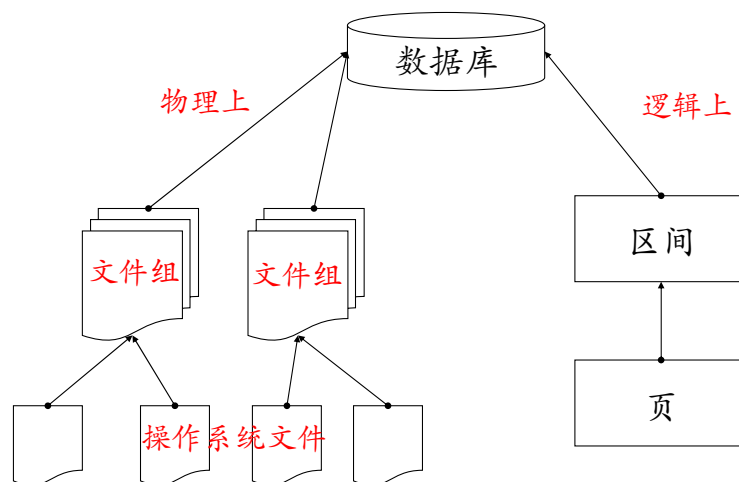
图 11.6: 数据库存储结构
