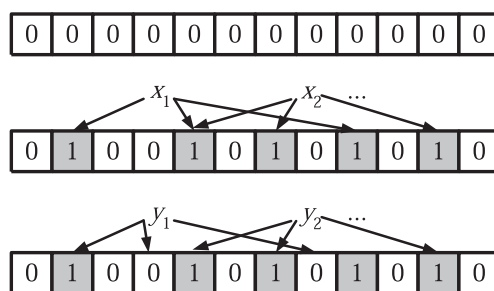
图 11.20: Bloom Filter 的一个例子
