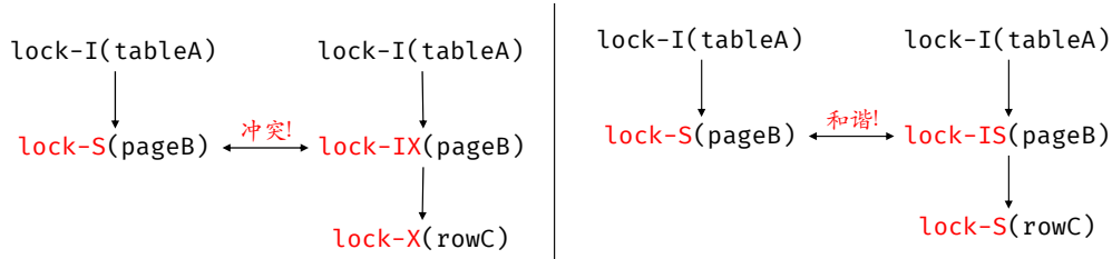
图 9.4: 意向锁 I 的细化
