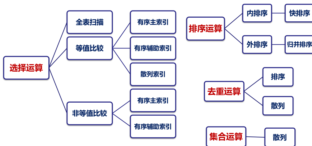
图 12.3: 实现各种逻辑运算的物理算子概览
