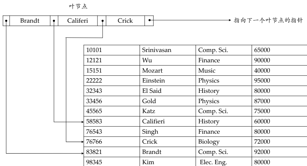
图 11.9: B+ 树的叶节点
