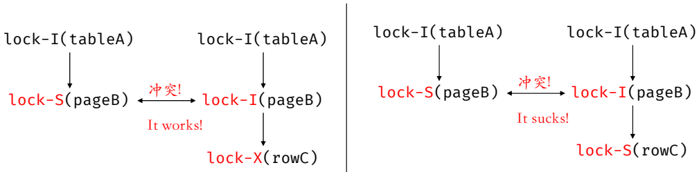
图 9.3: 意向锁 I 的不足之处
